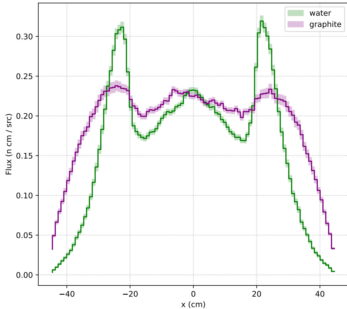
Thermal neutrons
